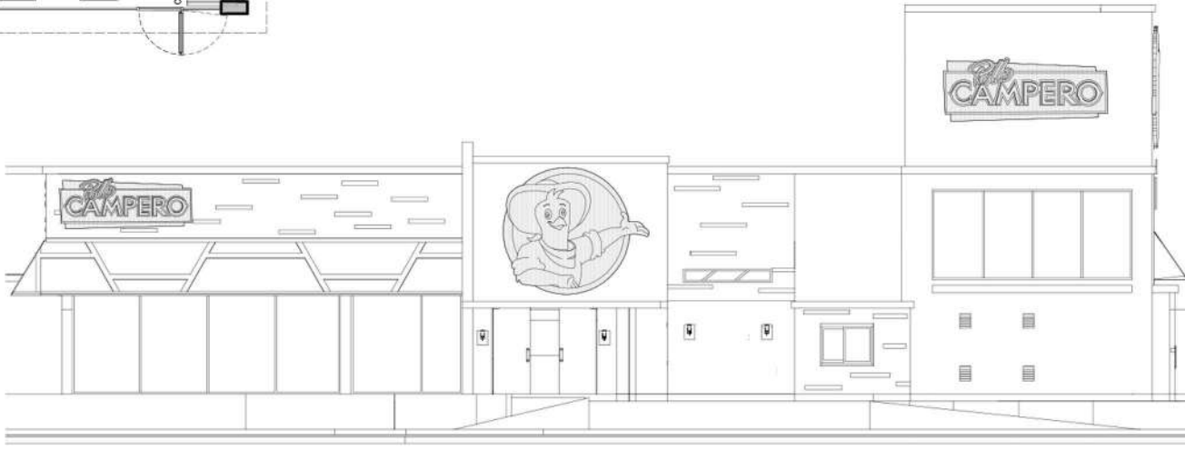
FACHADA FRONTAL
